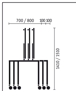
Objekttische (Seitenansicht)
